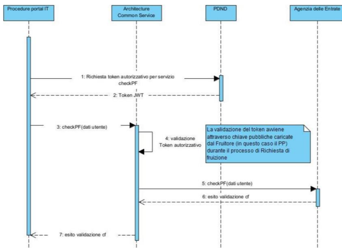
Figura 14 - Integrazione tra PP e ACS SDG IT per servizio checkPf
