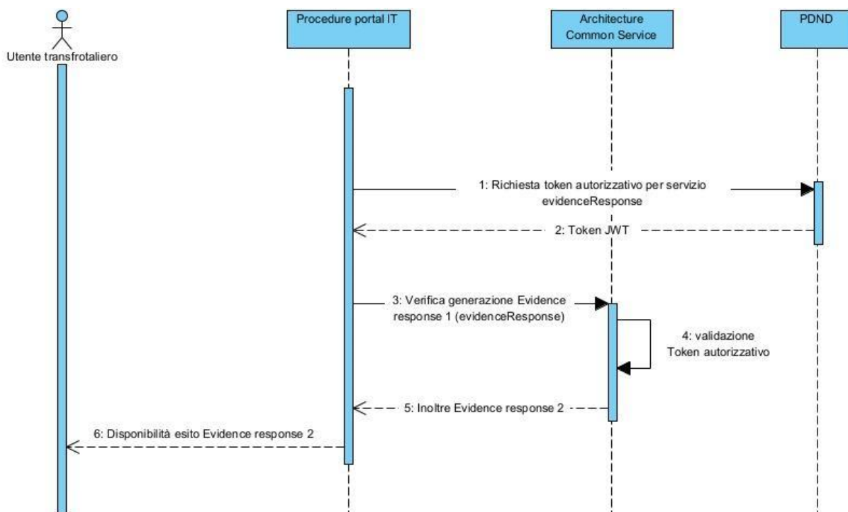
Figura 13 - Interazione tra PP e ACS SDG IT per recupero Evidence Response 2
