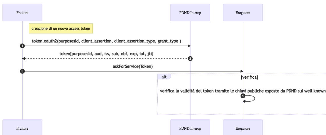
Figura 4 - Richiesta di un access token e fruizione del servizio
