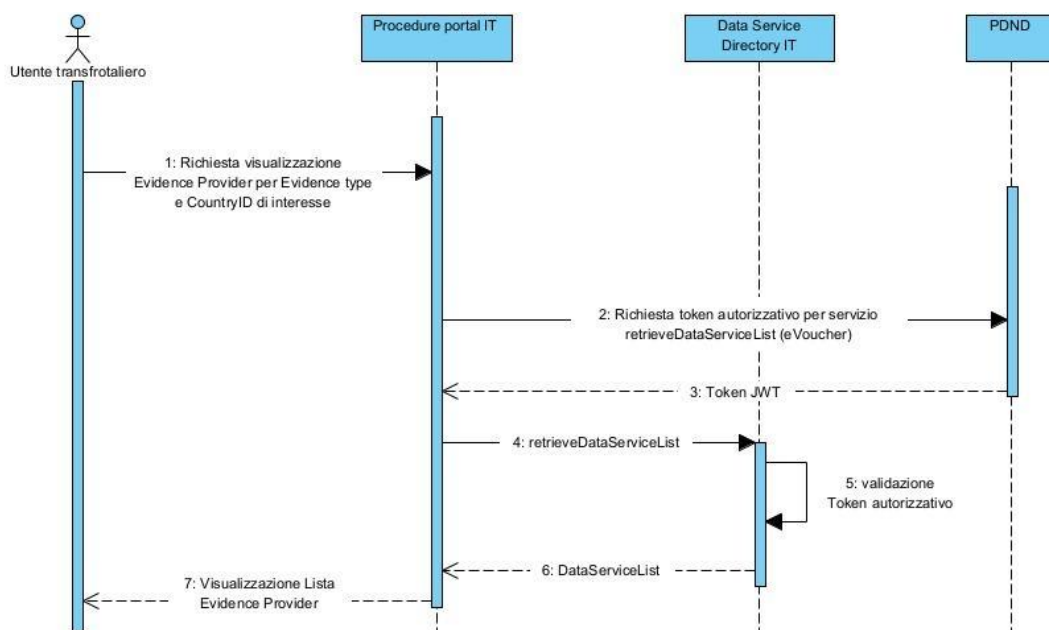
Figura 9 - Interazione tra PP e DSD per recupero lista dei data service
