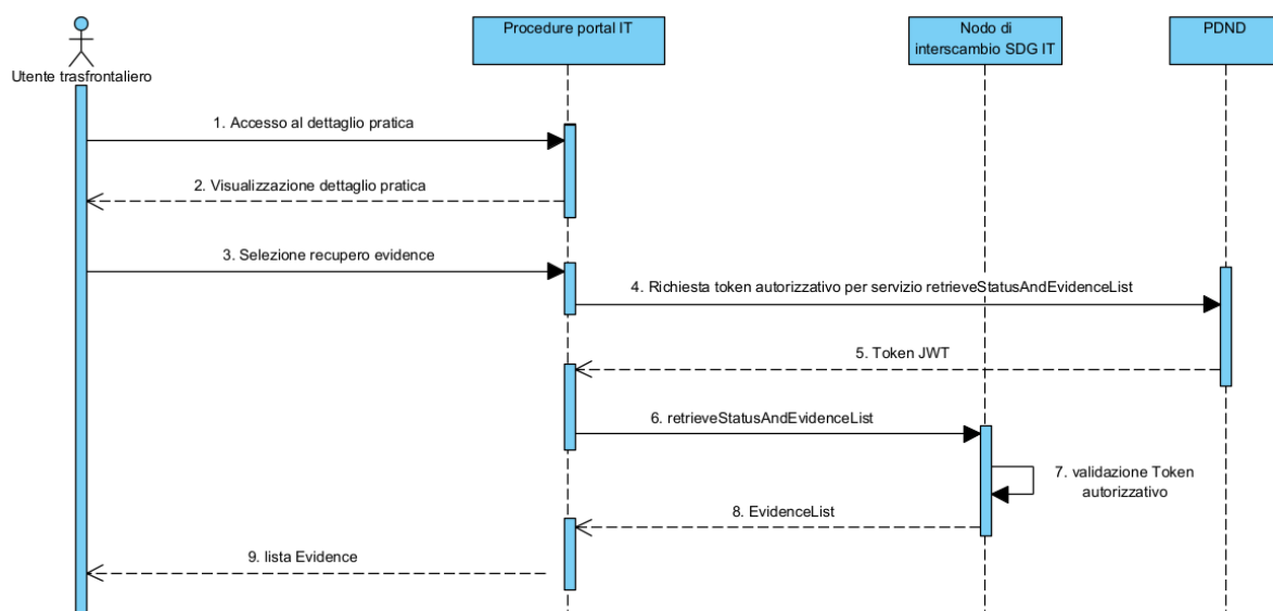
Figura 19 - Interazione tra PP e Nodo di interscambio SDG IT per retrieveStatusAndEvidenceList
