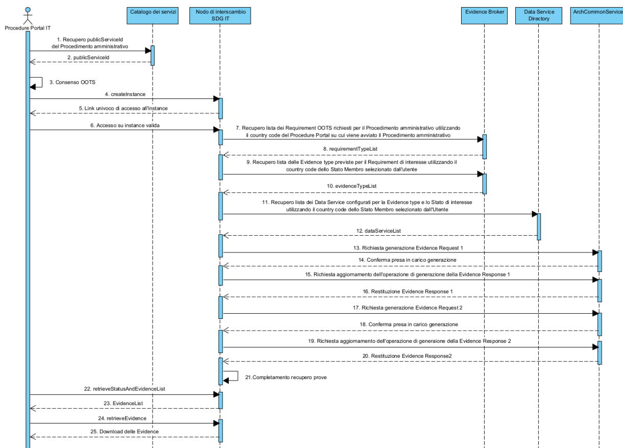
Figura 17 - Interazione previste tra PP IT, Nodo di interscambio SDG IT e Componenti Nazionali SDG IT
