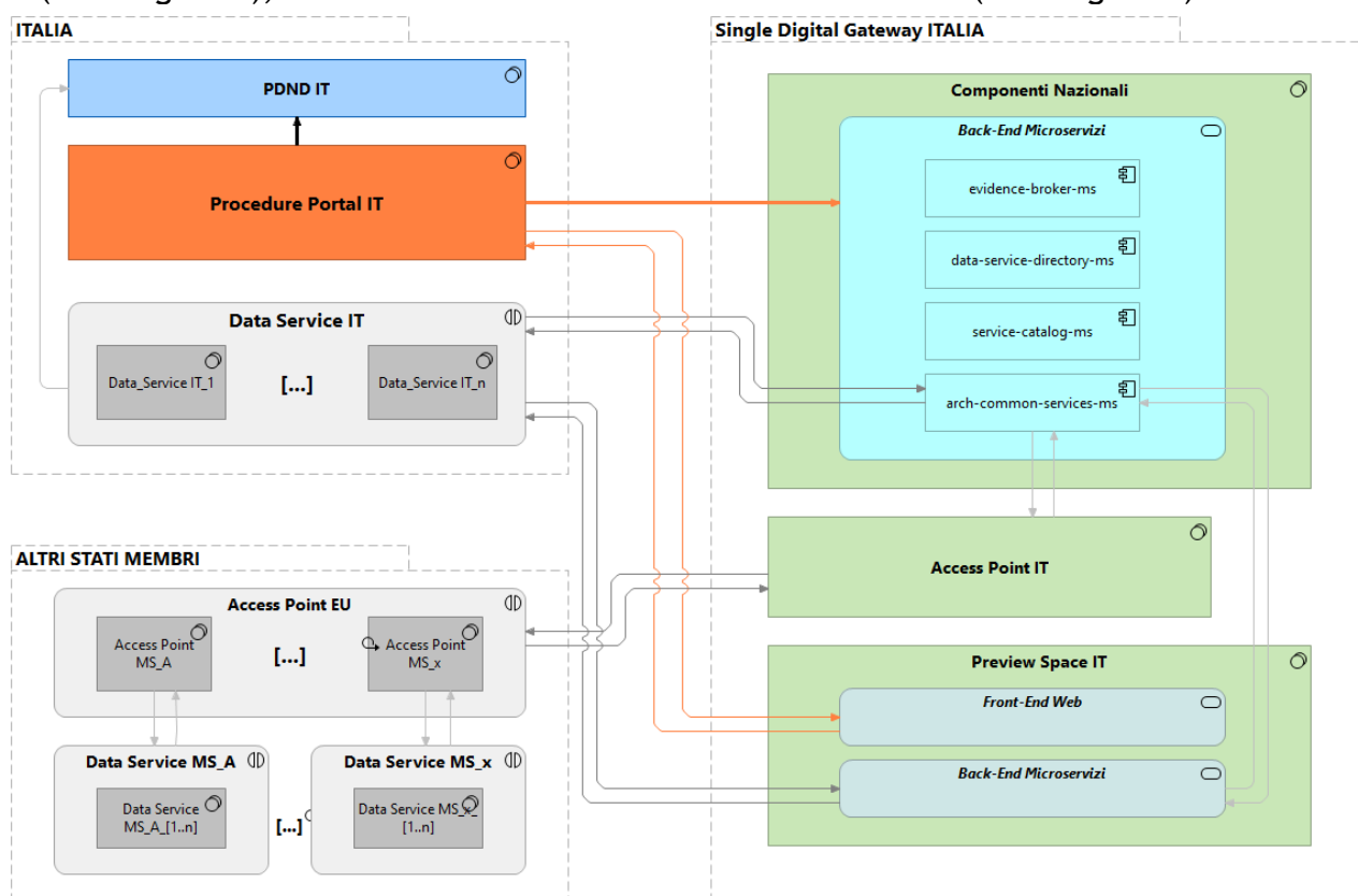
Figura 1 - Diagramma logico dell'infrastruttura SDG IT e degli attori esterni coinvolti in caso di interazione diretta con i Componenti nazionali SDG IT
