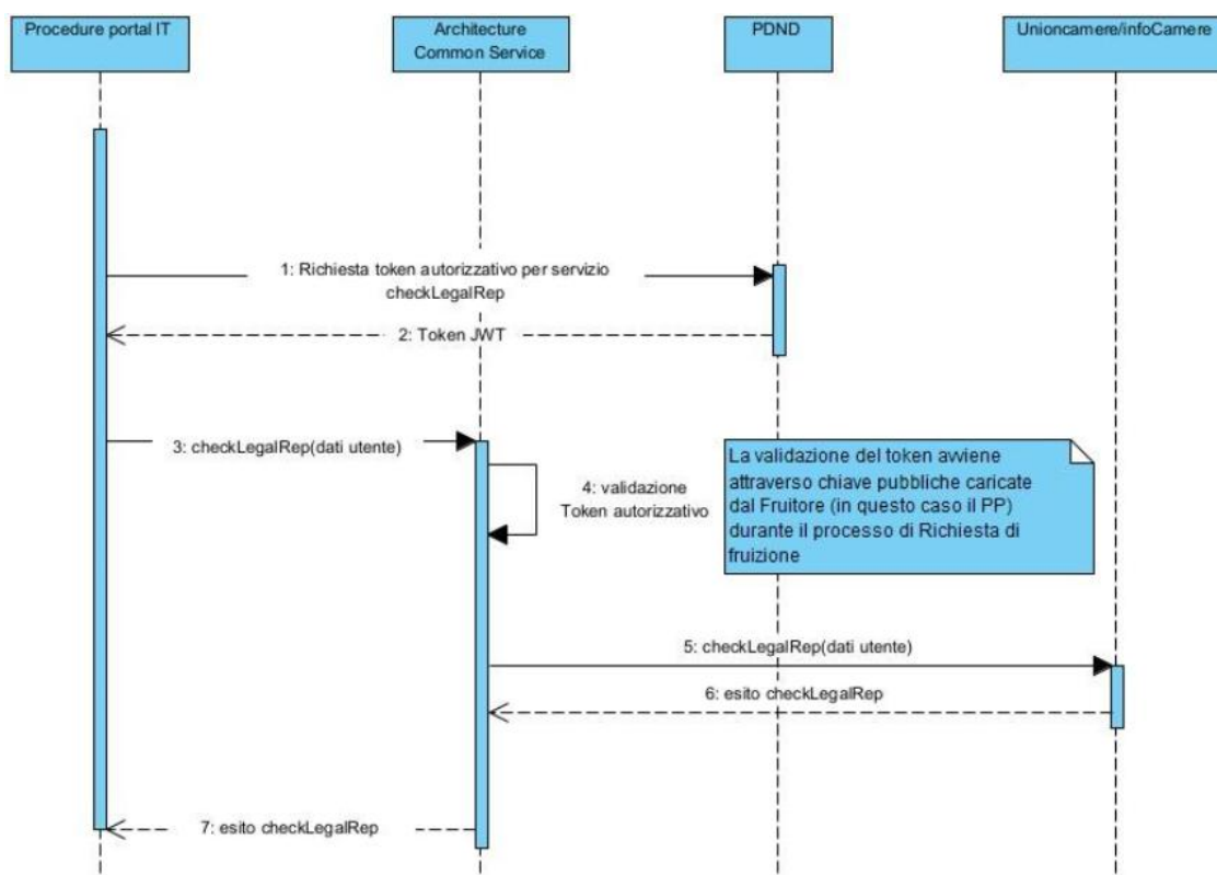
Figura 16 - Integrazione tra PP e ACS SDG IT per servizio checkLegalRep
