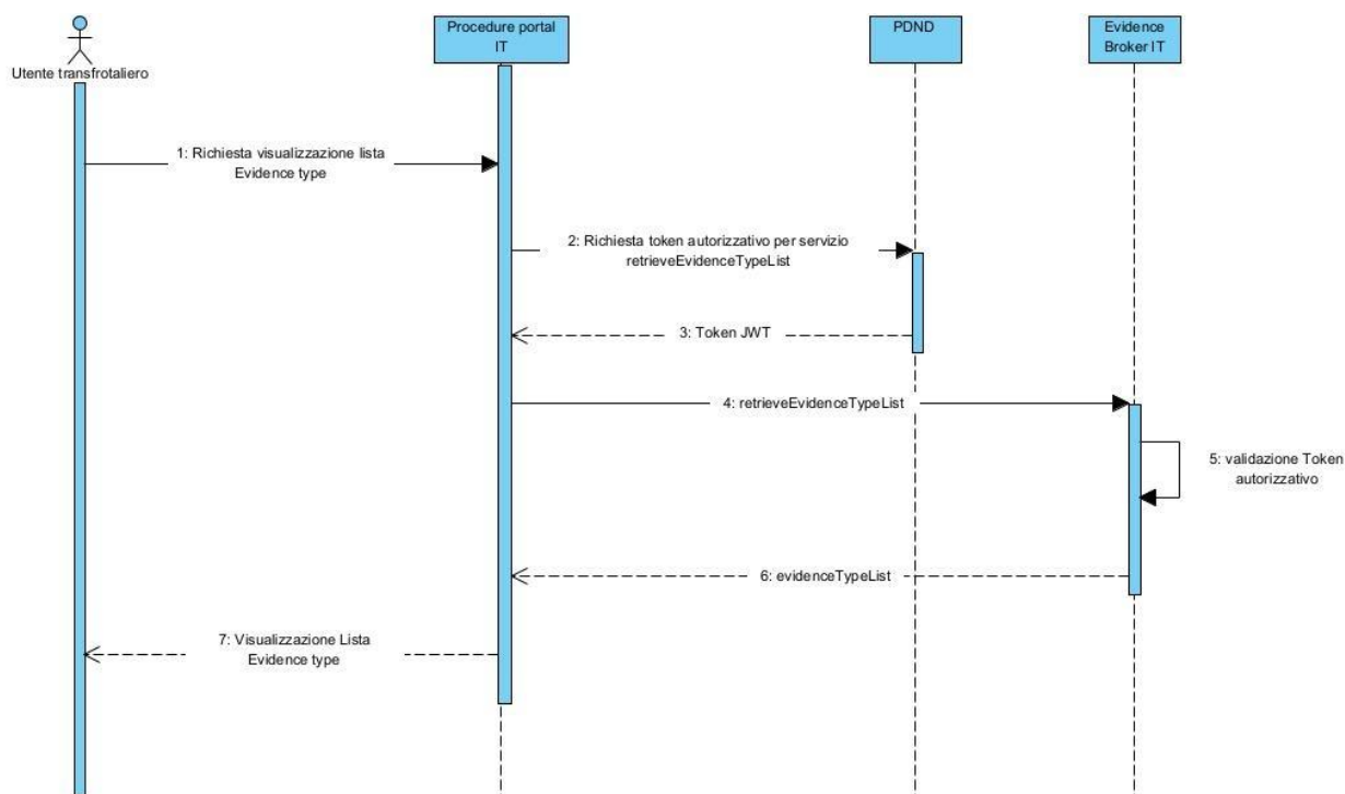
Figura 8 - Interazione tra PP ed EB per recupero lista di Evidence type
