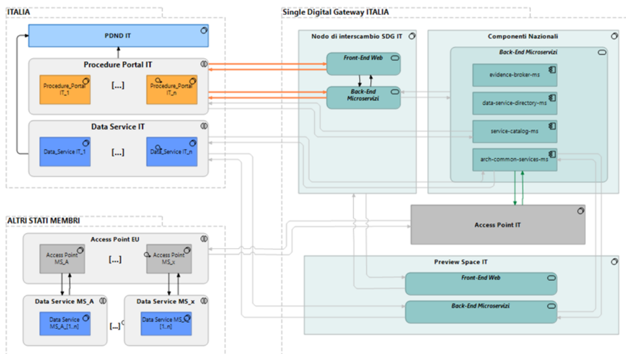
Figura 2 - Diagramma logico dell'infrastruttura SDG IT e degli attori esterni coinvolti in caso di interazione tramite Nodo di interscambio SDG IT
