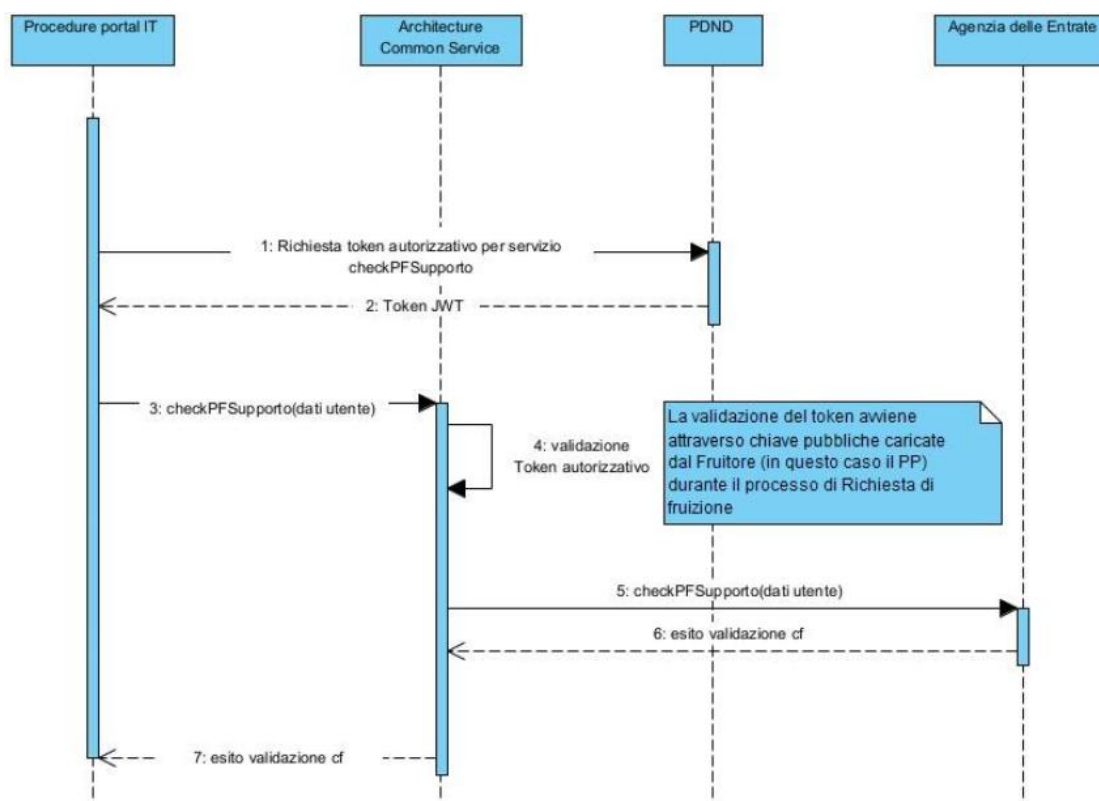
Figura 15 - Integrazione tra PP e ACS SDG IT per servizio checkPfSupporto
