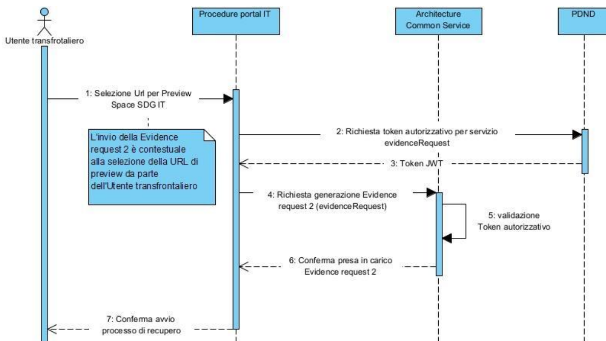
Figura 12 - Interazione tra PP e ACS SDG IT per invio Evidence Request 2
